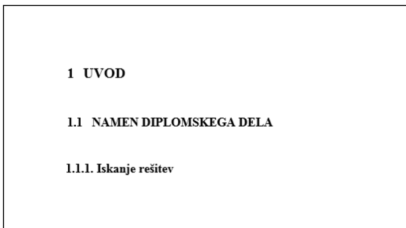
Slika 8: Oblike slogov
