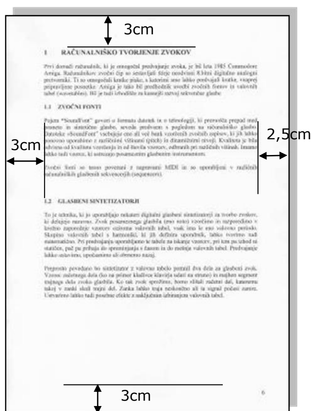
Slika 1: Nastavitev robov
