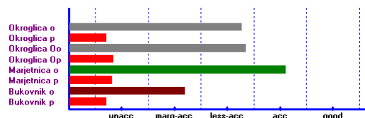
Slika 1: Rezultati vrednotenja
